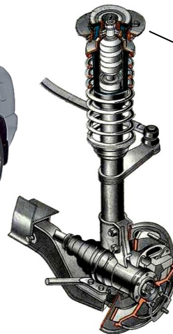
Передняя подвеска
