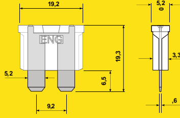
BIÇAK SİĞORTA BLADE FUSE
