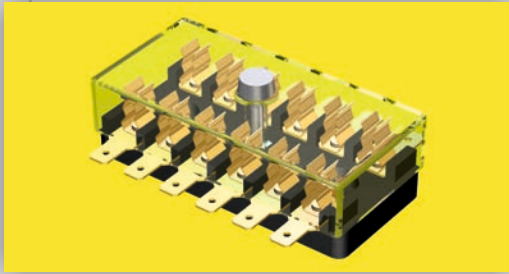
26 0127 MASSEY FERGUSON SİGORTA KUTUSU
