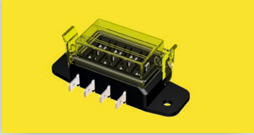
26 0610 4'LÜ SİGORTA KUTUSU YANDAN ÇIKIŞLI TERMİNALİ
