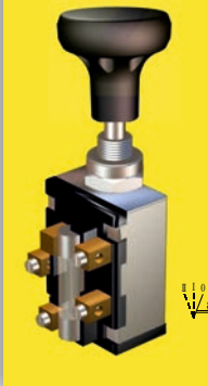
01 0502 ÇİFT ÇEKME Lİ ANAHTAR 20 A SİGORTALI HEADLIGHT PUSH-PULL SWITCH (20 A FUSE)
