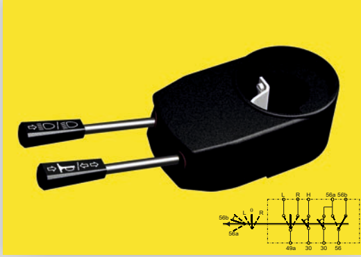
34 0512 50 NC SİNYAL KOLU
