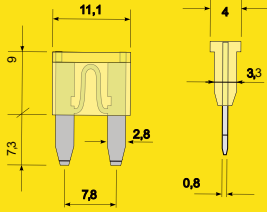
MINI BIÇAK SİĞORTA MINI BLADE FUSE
