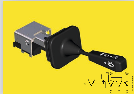
34 0527 MAGIRUS SİLECEK KOLU
