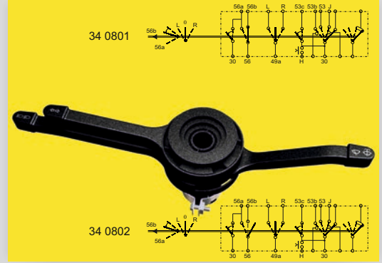
34 0801 TOFAŞ 131SİNYAL KOLU Y.M.
