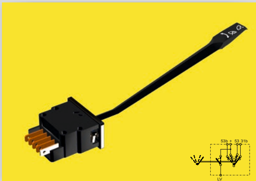
01 1520 RENAULT SU SİLGİ KOLU
