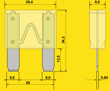
MAXI BIÇAK SİĞORTA MAXI BLADE FUSE
