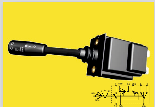
34 0530 TRAKTÖR SİNYAL KOLU
