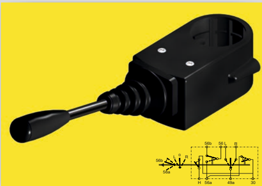
34 0524 STAYR SİNYAL KOLU
